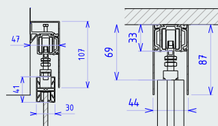
Coupe verticale en applique
