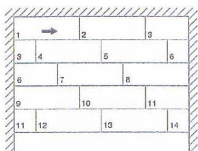
Figure 7 Pose des plaques de sol
